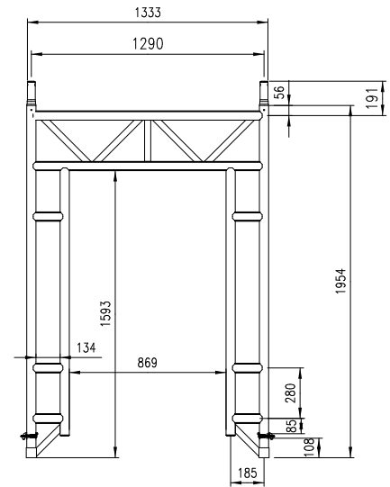
Basisdoorloopframe RS TOWER 52
