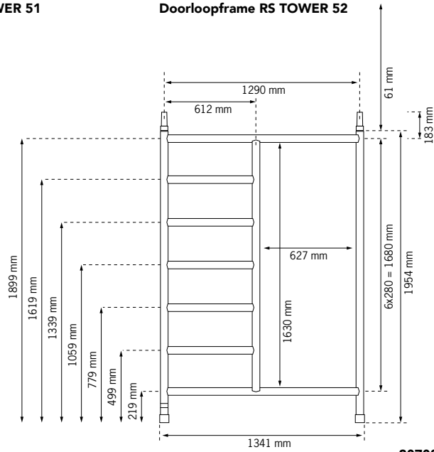
Doorloopframe RS TOWER 52
