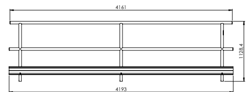
331624 Leuning DRB 4 m
